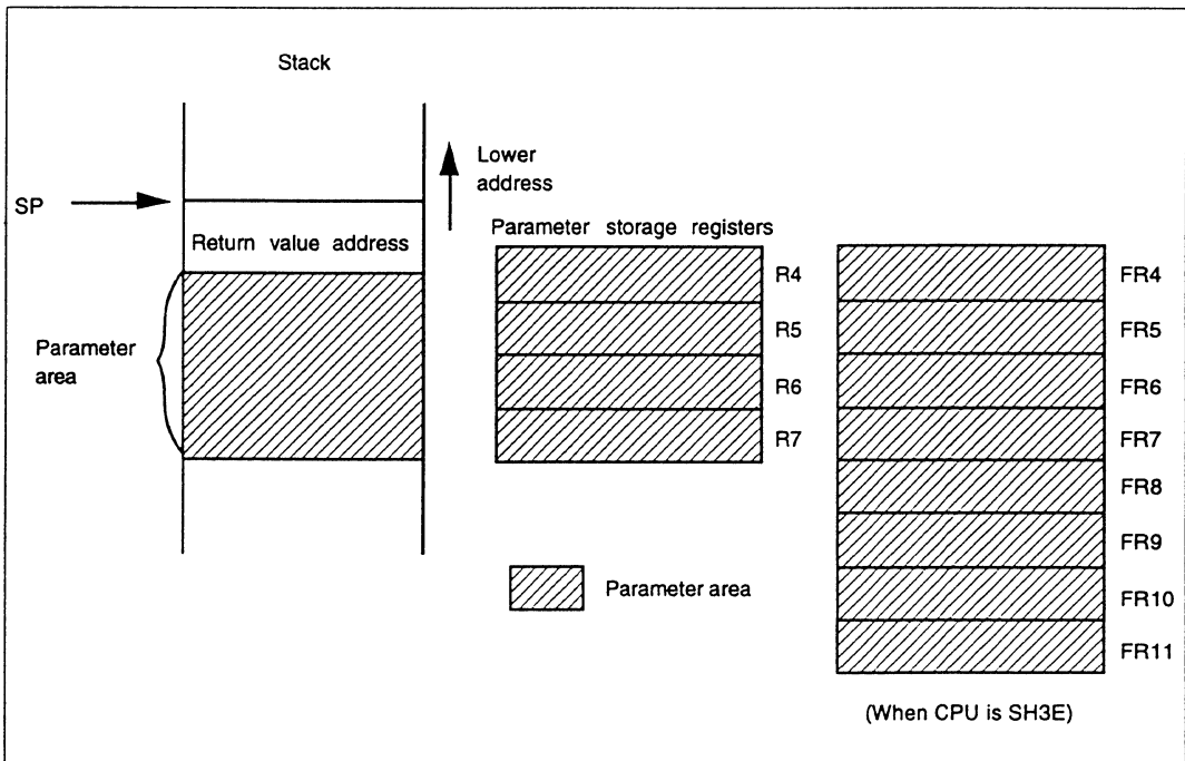
Figure 2.2 Parameter Area Allocation
